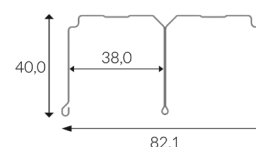
vrchná koľajnica
